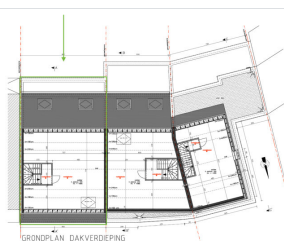
GRONDPLAN DARVERDIEPING
